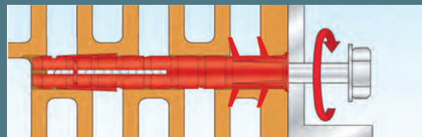
4. Заверните шуруп
